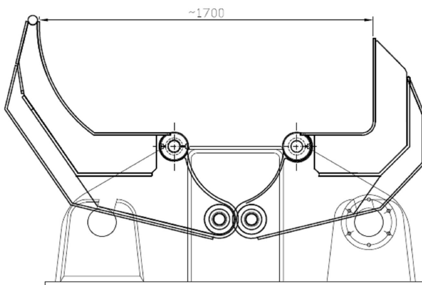
Schemat nr 3: widok na klapy górne
