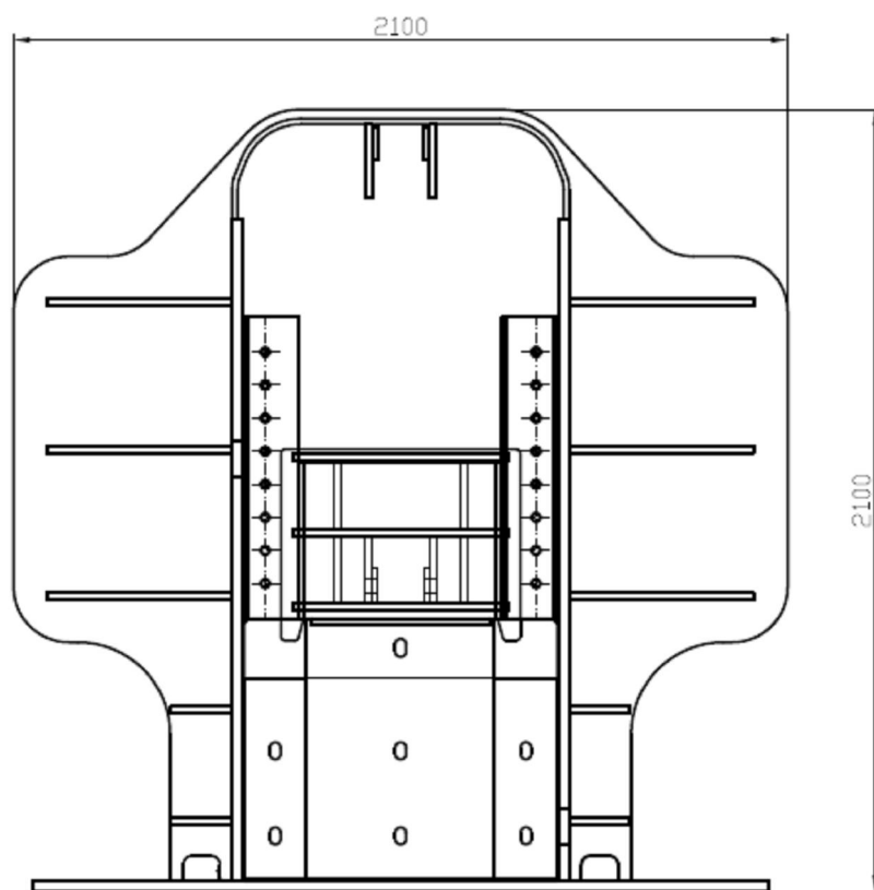
Schemat nr 2: widok paczkarki od frontu
